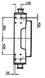
ANSICHT 1
